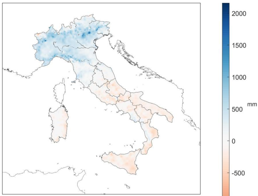
Figura 5.5: Anomalia della precipitazione cumulata annuale 2024, espressa in mm, rispetto al valore normale 1991-2020.
