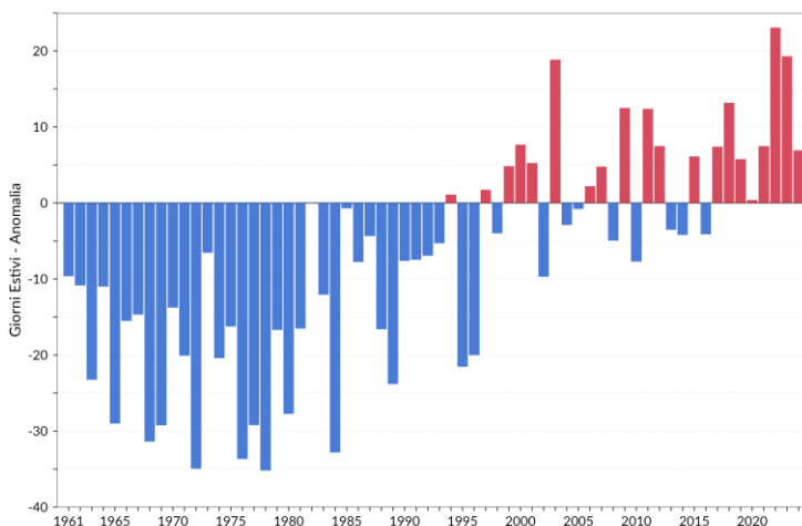
Figura 3.14: Serie delle anomalie medie annuali del numero di giorni estivi 12 in Italia rispetto al valore normale 1991-2020.
