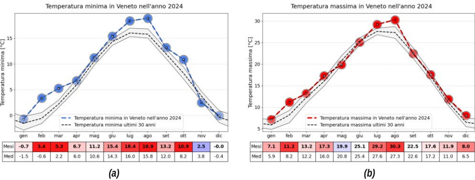
Figura 4: Medie mensili delle temperature minime (a) e delle temperature massime (b) nel corso del 2024. Il confronto con i percentili della climatologia 1991-2020 evidenzia: per la temperatura minima (a) 1 mese sotto al 25° percentile (novembre), nessun mese tra il 25° e il 50° percentile, 4 mesi tra il 50° e il 75° percentile (gennaio, aprile, maggio e dicembre) e 7 mesi oltre il 75° percentile (giugno, settembre, ...) di cui ben cinque oltre il 90° percentile (febbraio, marzo, luglio, agosto e ottobre); per la temperatura massima (b) nessun mese sotto al 25° percentile, 2 mesi tra il 25° e il 50° percentile (maggio e giugno), 1 mese al 50° percentile (settembre), 3 mesi tra il 50° e il 75° percentile (marzo, ottobre e novembre) e 6 mesi oltre il 75° percentile (gennaio, aprile, luglio, dicembre, ...) di cui 2 oltre il 90° percentile (febbraio e agosto).
