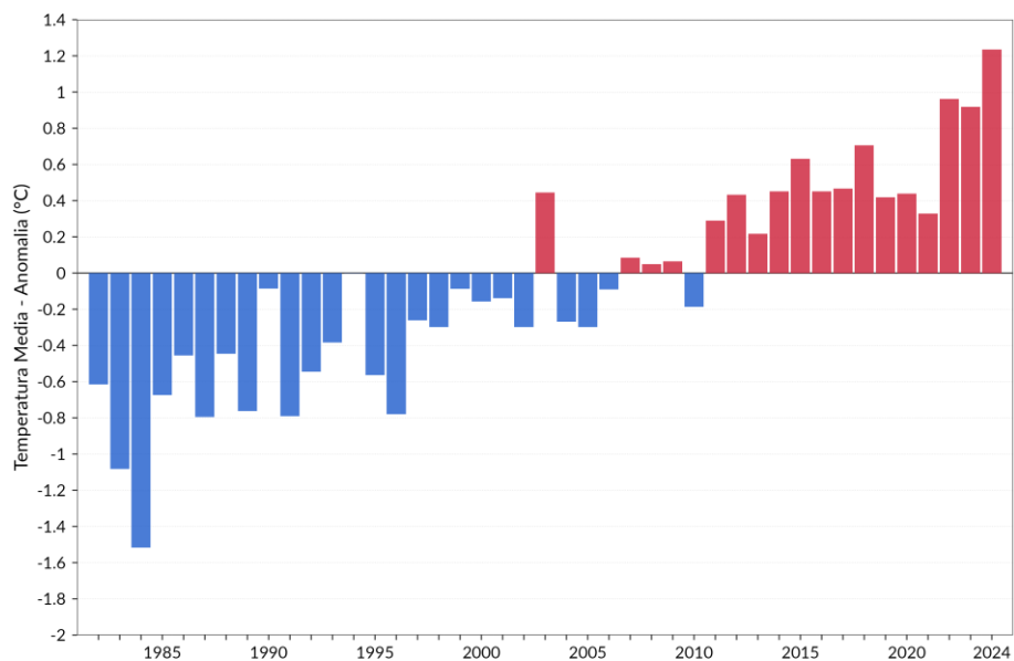
Figura 4.5: Serie delle anomalie medie annuali della temperatura media superficiale dei mari italiani, nell'intervallo 1982-2024, rispetto al valore normale 1991-2020.
