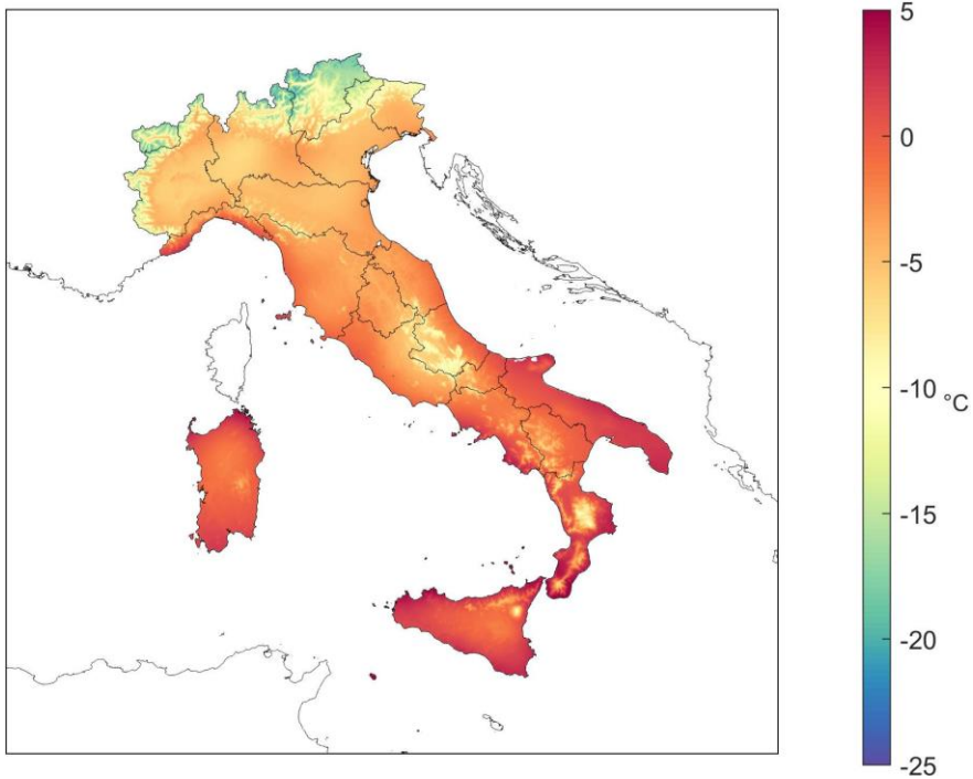
Figura 3.2: Temperatura minima assoluta 2024.
