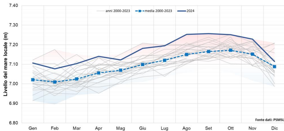
Figura 4. Almeria (Andalusia). Confronto tra valori mensili 2024 e medie nel periodo 2000-2023 per il livello del mare.
