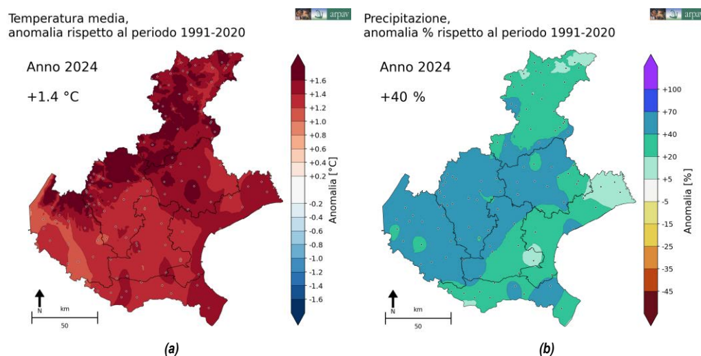
Figura 2: Carte dell'anomalia in °C della temperatura media annuale del 2024 rispetto alla norma del periodo 1991-2020 sul Veneto (a) e dell'anomalia percentuale della precipitazione cumulata annuale del 2024 rispetto alla norma del periodo 1991-2020 sul Veneto (b).
