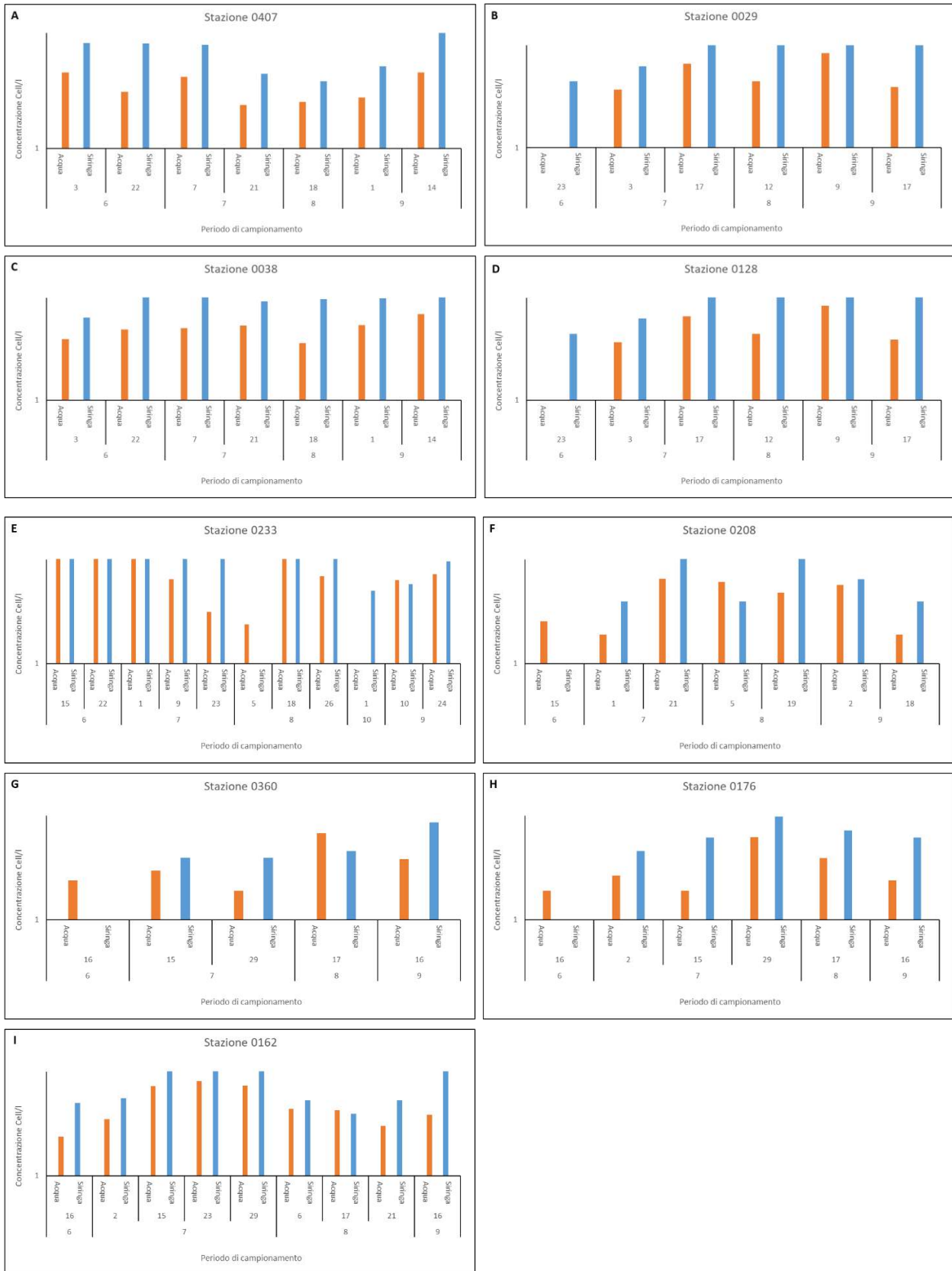
Grafico 1: Confronto tra le concentrazioni di O. cf. ovata nei campioni di acqua e di siringa. A-D stazioni nell'area della Città metropolitana di Roma; E-I stazioni della provincia di Latina (■ cell/l acqua; ■ cell/l siringa).
