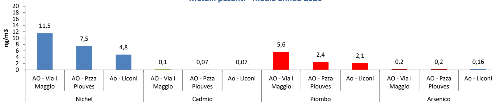
Metalli pesanti - media annua 2020
