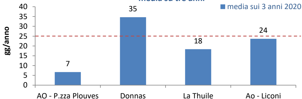
N di giorni di superamento dell'obiettivo a lungo termine: 120 µg/m 3 da non superare per più di 25 v. per anno civile come media su tre anni
