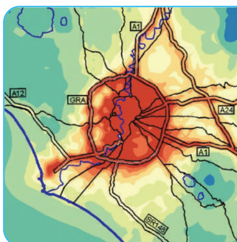
NO 2 – media annua 2018 dominio di Roma (1 km x 1 km)
