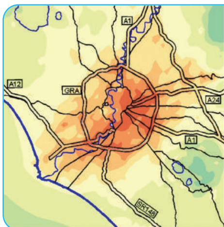
\text{PM}_{25} : media annua 2018 dominio di Roma (1 km x 1 km)
