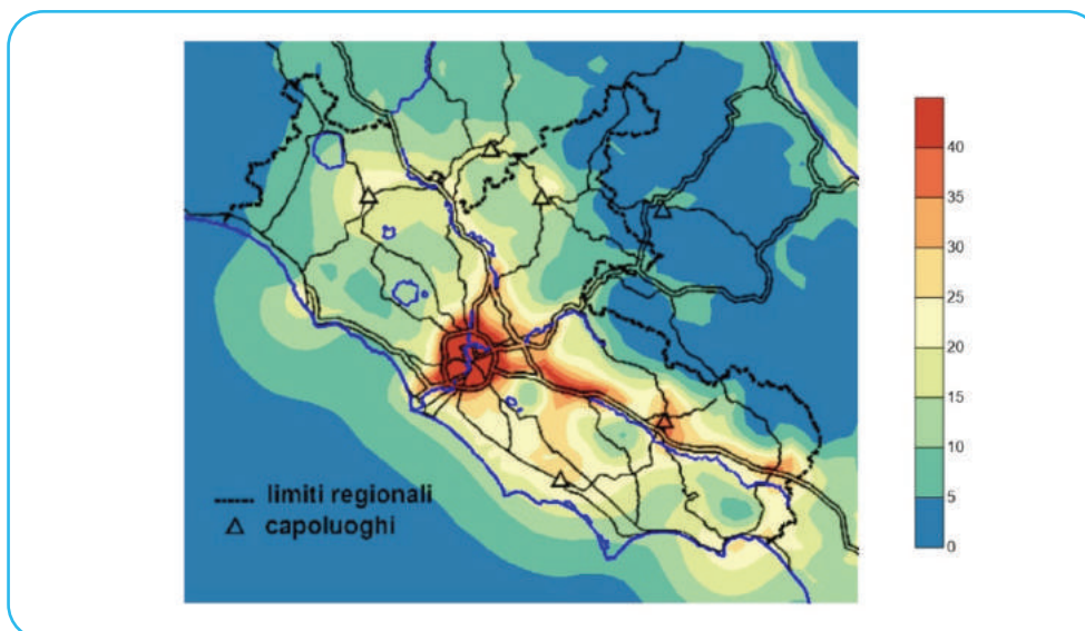
NO 2 – media annua 2018 dominio di Roma (1 km x 1 km)
