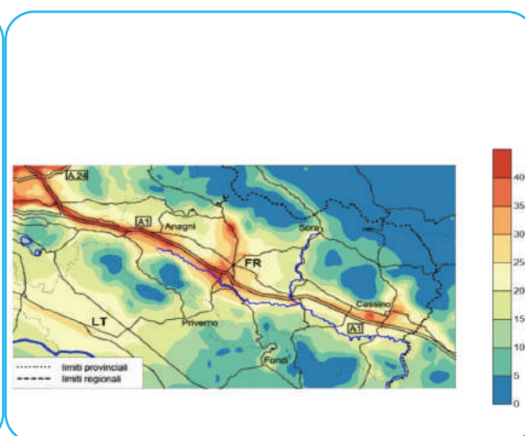
NO 2 – media annua 2018 dominio Valle del Sacco (1 km x 1 km)
