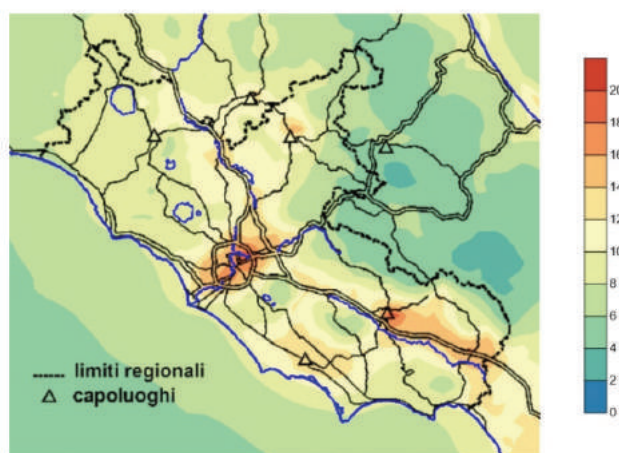
\text{PM}_{25} : media annua 2018 dominio di Roma (1 km x 1 km)
