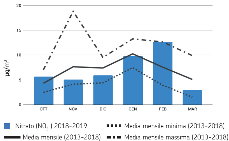
Nitrato, stazione Rimini Marecchia, ottobre 2018 - marzo 2019
