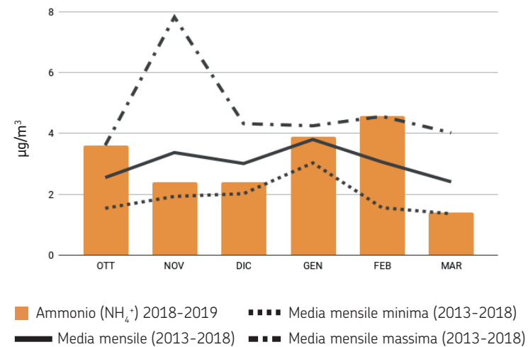
Ammonio, stazione Rimini Marecchia, ottobre 2018 - marzo 2019
