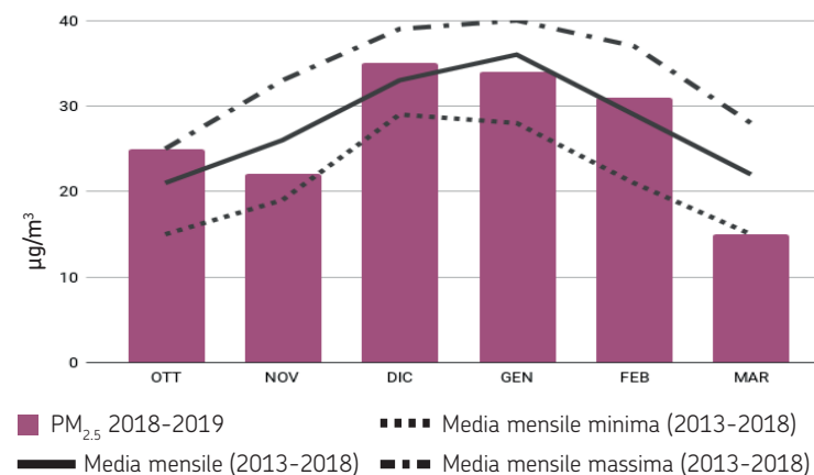
PM 2.5 PM 2.5 stazione Bologna Gobetti, ottobre 2018 - marzo 2019
