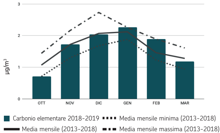
Carbonio elementare, stazione Rimini Marecchia, ottobre 2018 - marzo 2019
