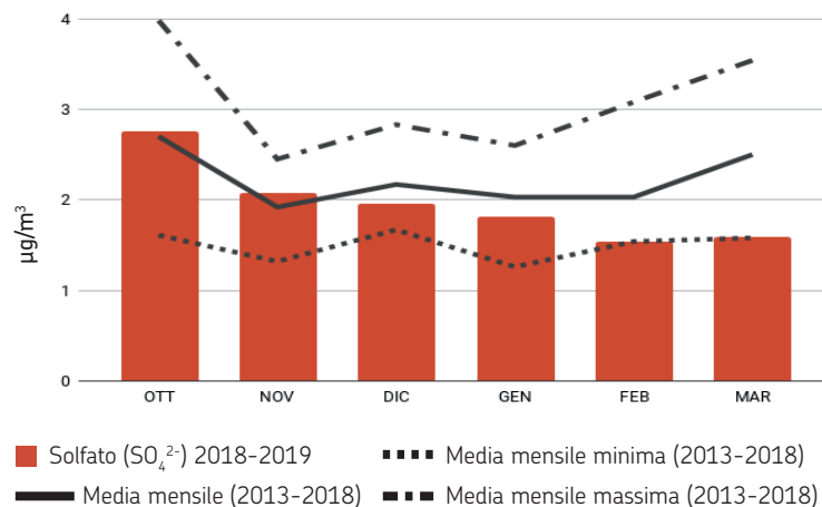
Solfato, stazione Parma Cittadella, ottobre 2018 - marzo 2019
