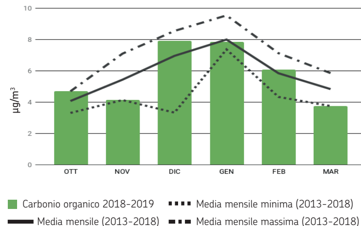
Carbonio organico, stazione Bologna Gobetti, ottobre 2018 - marzo 2019
