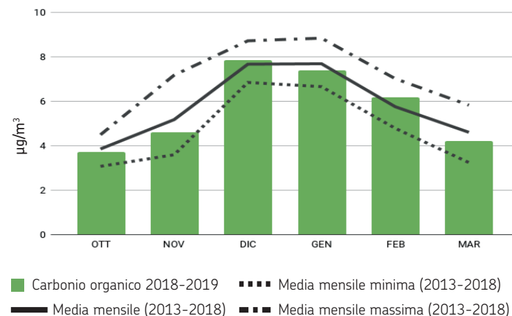
Carbonio organico, stazione Parma Cittadella, ottobre 2018 - marzo 2019
