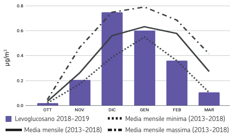
Levoglucosano nella stazione Bologna Gobetti, ottobre 2018 - marzo 2019
