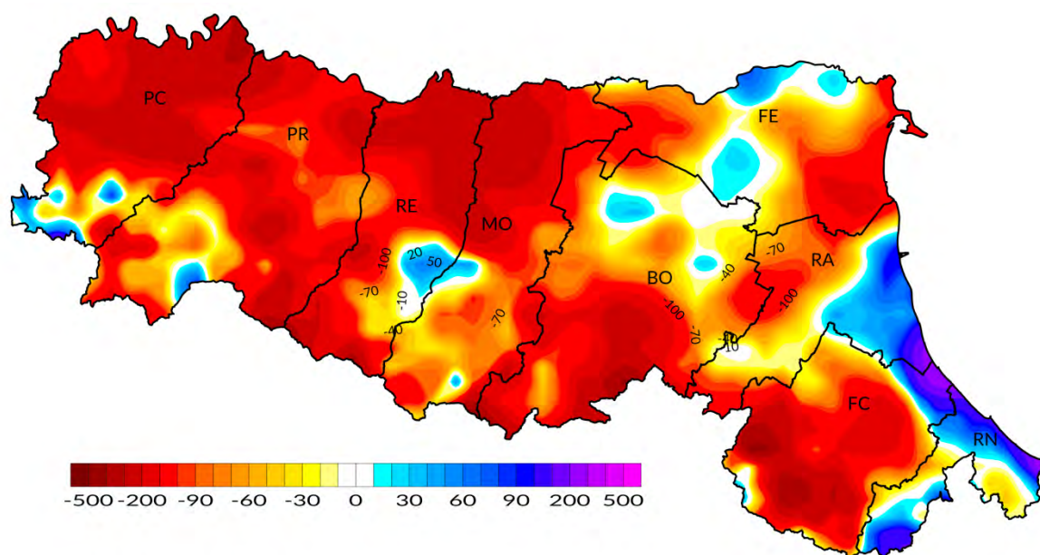
Figura 25: anomalia del bilancio idroclimatico annuo 2018 (mm) rispetto al clima 1961-1990.
