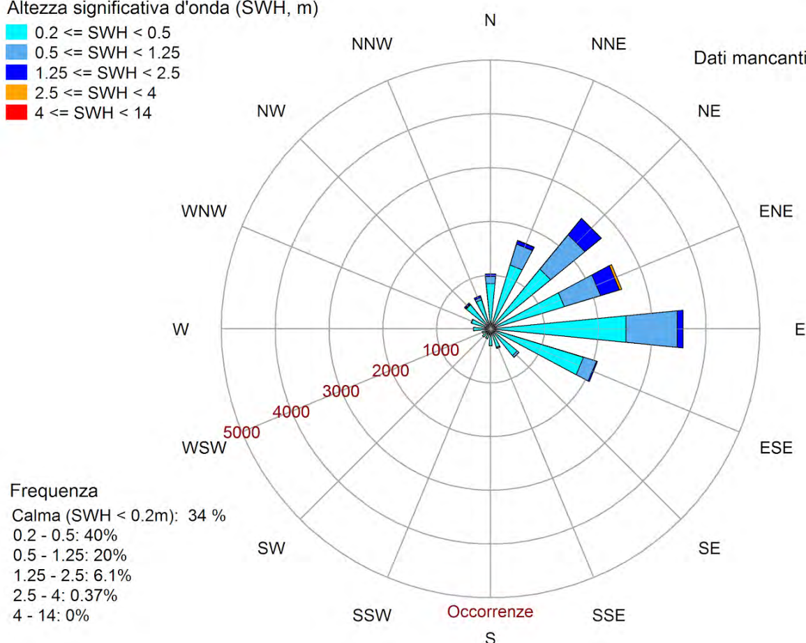
Figura 1: rosa delle onde registrate dalla boa ondametrica di Cesenatico (FC) nell'anno 2018
