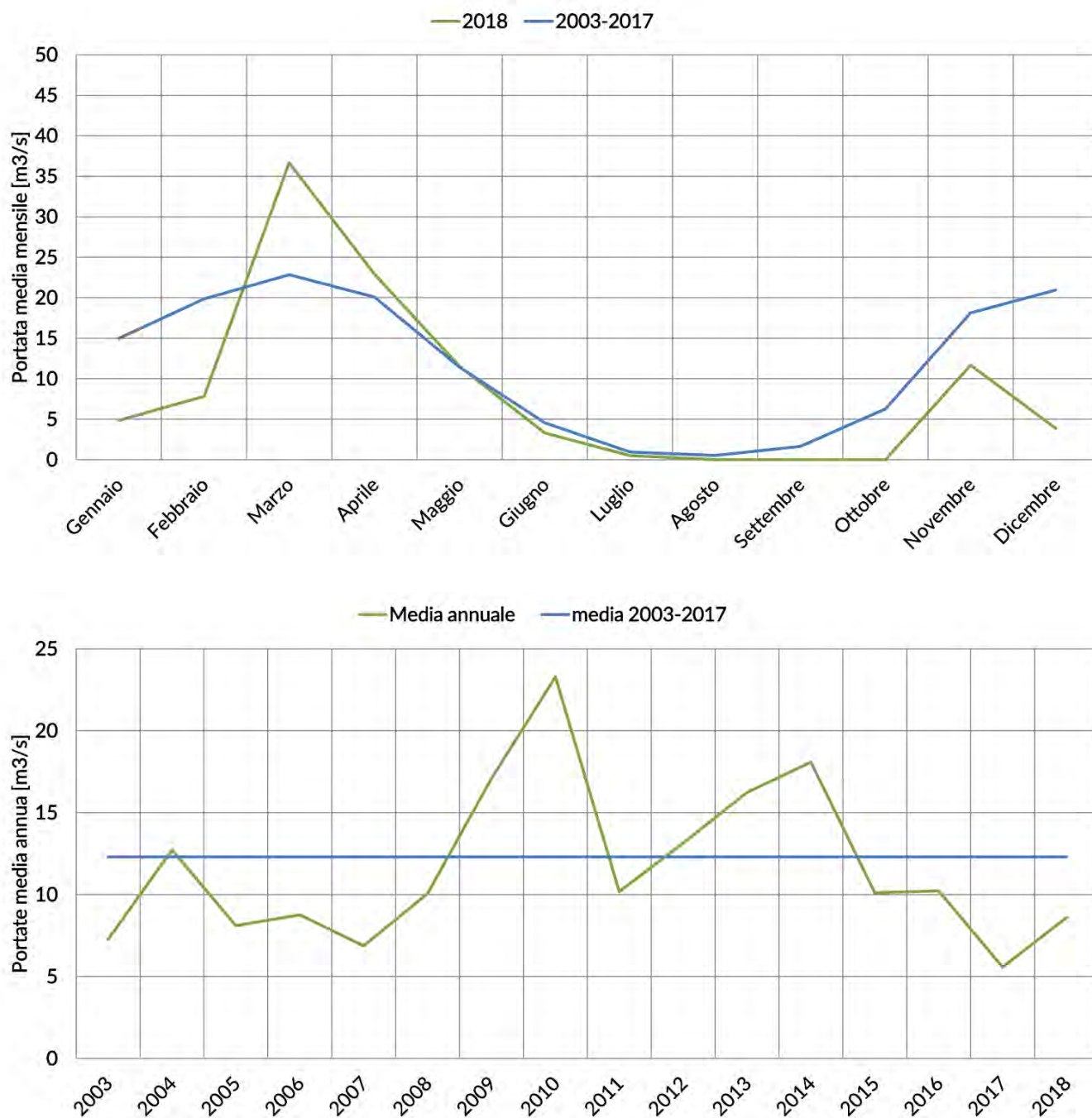
Figura 3. Torrente Parma, sezione idrometrica di Parma Ponte Verdi, bacino sotteso di 600 km 2 . In alto le portate medie mensili del 2018 e i corrispondenti valori medi 2003-2017. In basso le portate medie annuali dal 2003, e la media generale 2003-2017.
