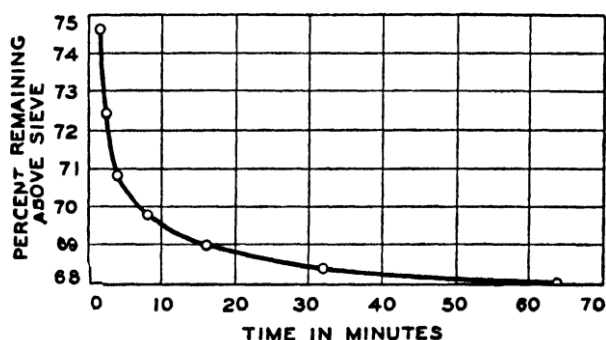
Figura 8. Progressione temporale della setacciatura (Krumbein & Pettjohn, 1938).
