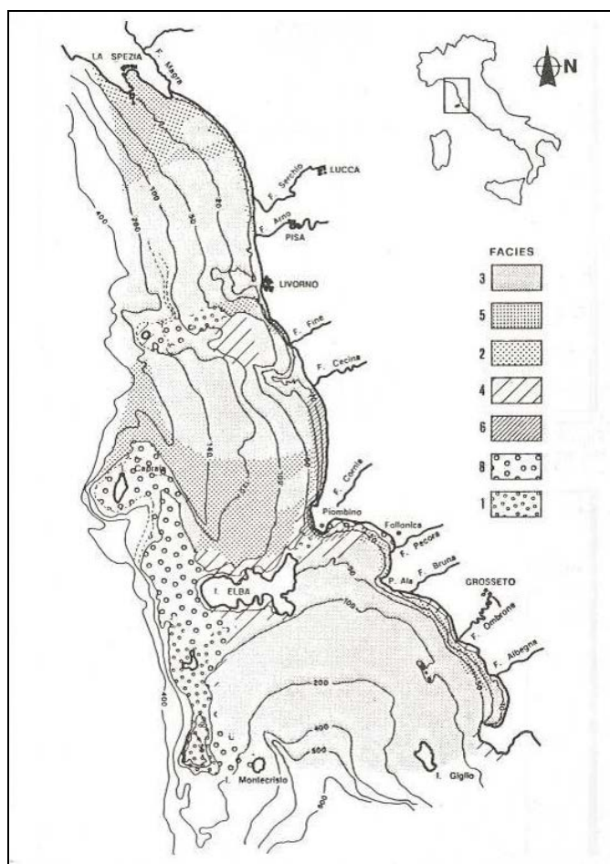
Figura 2. Distribuzione areale delle facies granulometriche dell'area toscana (De Simone et al., 1993). Legenda: 1) ghiaia e sabbia grossolana; 2) sabbia pelitica; 3) argilla; 4) limo; 5) limo sabbioso; 6) sabbia medio-fine; 8) sabbia medio-grossolana.
