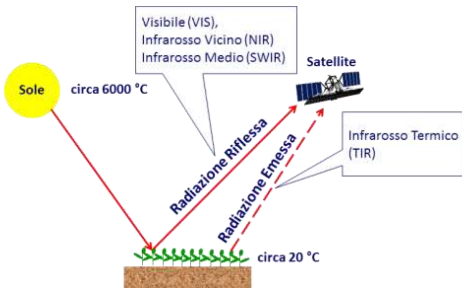
Figura 7. Un sensore passivo ottico (in questo caso a bordo in un satellite) può acquisire, in funzione della regione spettrale in cui opera, la radiazione elettromagnetica proveniente dal Sole e riflessa dalla superficie terrestre (oltre che dall'atmosfera) oppure la radiazione elettromagnetica emessa dalla superficie terrestre stessa. La radiazione riflessa è concentrata nelle regioni spettrali del visibile (VIS), infrarosso vicino (NIR) e infrarosso medio (SWIR). La radiazione emessa è concentrata nella regione spettrale dell'infrarosso termico (TIR).
