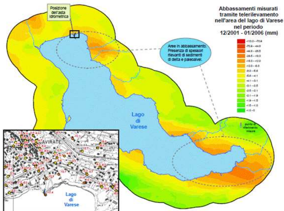
Figura 15. Esempio di utilizzazione della interferometria differenziale SAR per misurare la subsidenza delle sponde del lago di Varese nel periodo 2001-2006.
