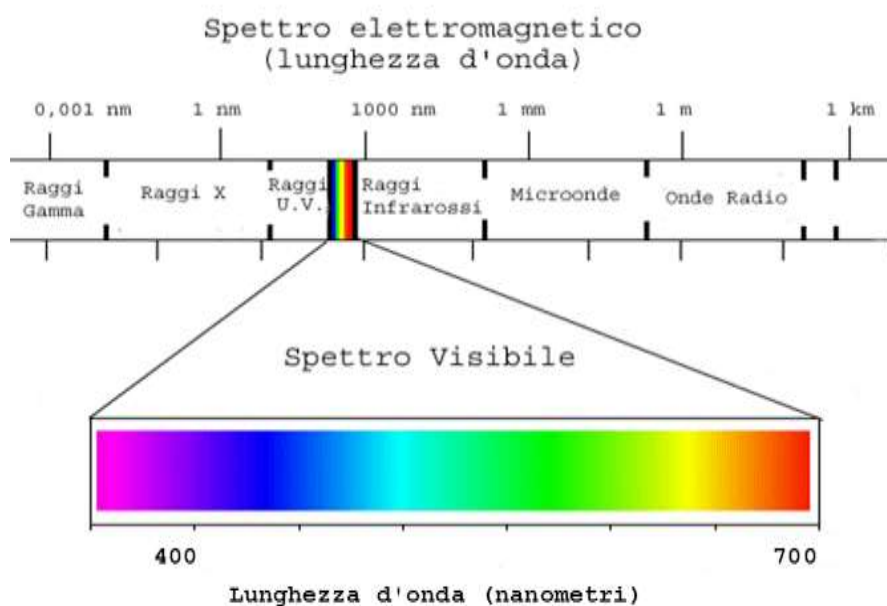
Figura 6. Spettro elettromagnetico in cui è evidenziata la regione del visibile.
