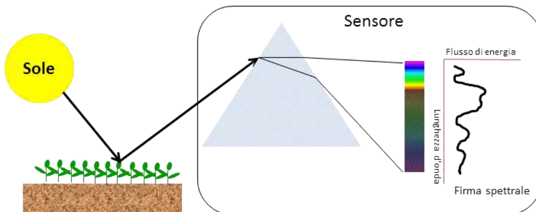
Figura 8. Gli oggetti presenti sulla superficie terrestre (in questo caso la vegetazione) riflettono parzialmente la radiazione elettromagnetica proveniente dal Sole. Un sensore ottico riceve la radiazione e la decompone in bande spettrali che consentono di ottenere la firma spettrale dell'oggetto osservato.
