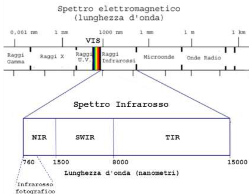
Figura 5. Spettro elettromagnetico in cui sono evidenziate le regioni del visibile (VIS), dell'infrarosso vicino (NIR), dell'infrarosso medio (SWIR) e dell'infrarosso termico (TIR).
