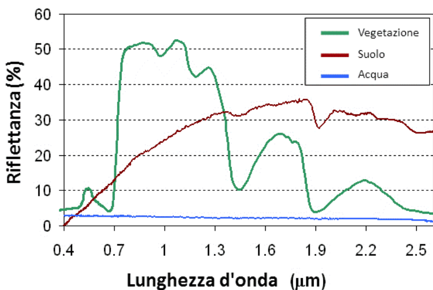
Figura 9. La misurazione della firma spettrale permette di discriminare tra loro gli oggetti presenti sulla superficie terrestre. Il diagramma presenta le firme spettrali tipo della vegetazione, del suolo e dell'acqua.
